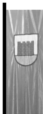
Hissflagge
